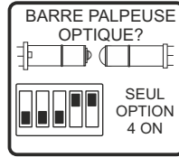
4. CONFIGURATION DU TYPE DE BARRE PALPEUSE (VOIR PARAGRAPHE 11.2)
